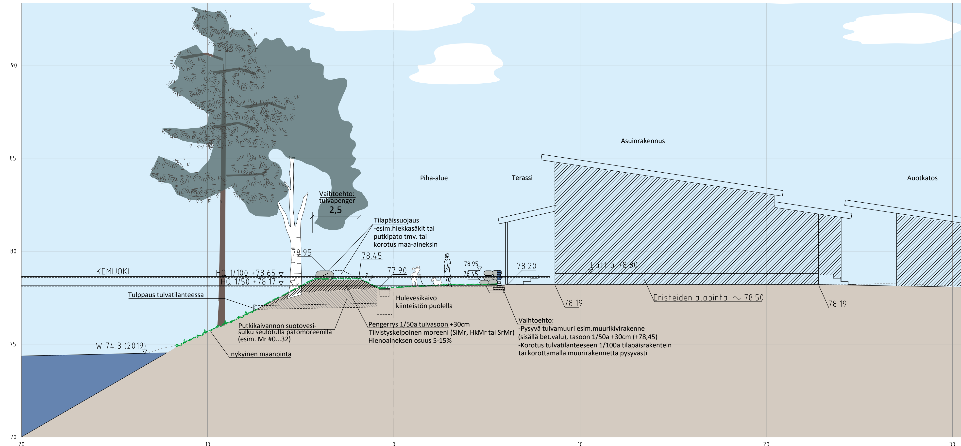
Leikkaus Kulpinranta PL230 / Kulpinranta 3-5 ja 7 1:100
