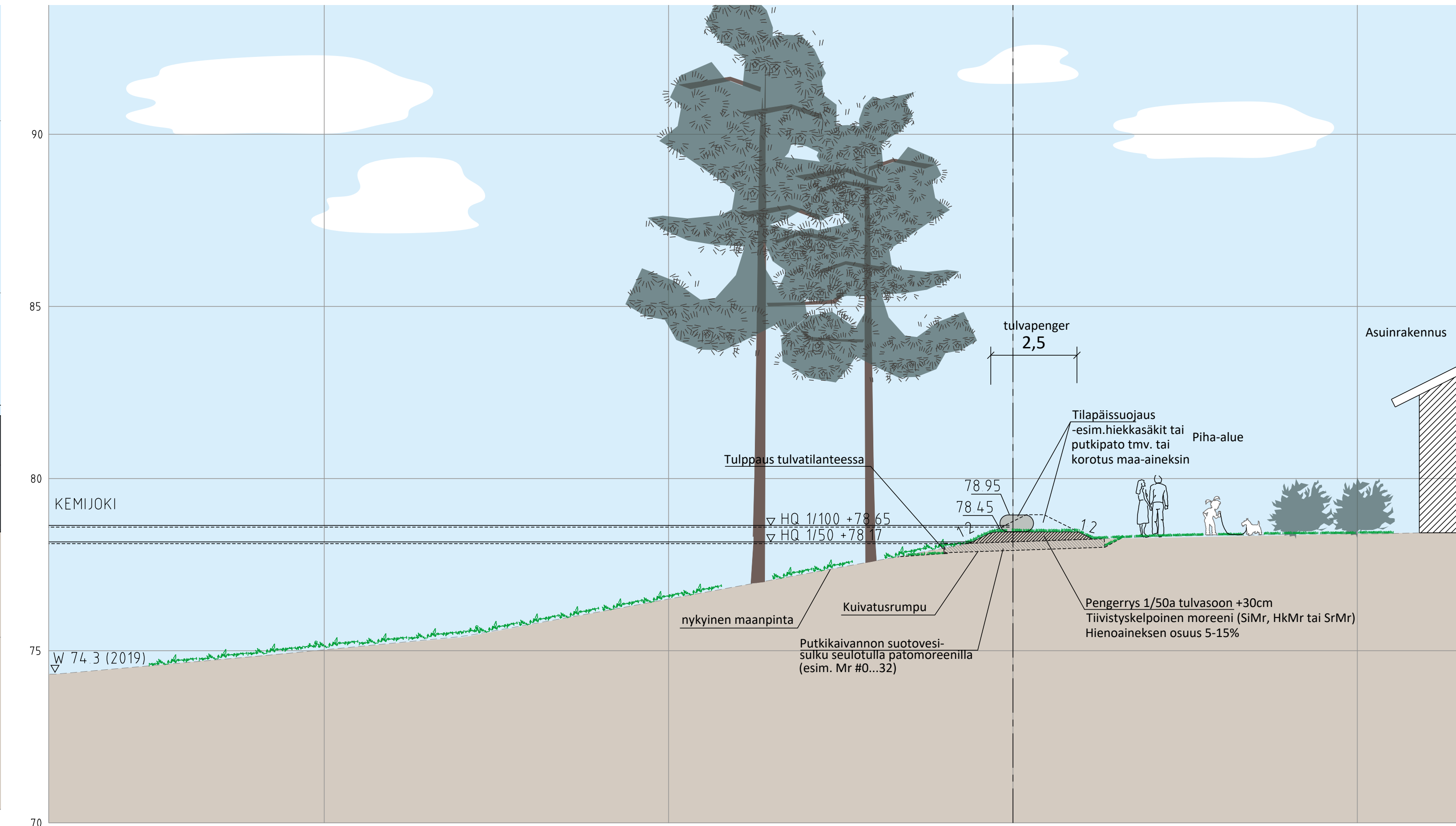
Leikkaus Kulpinranta PL746 / Sahatie 5 1:100
