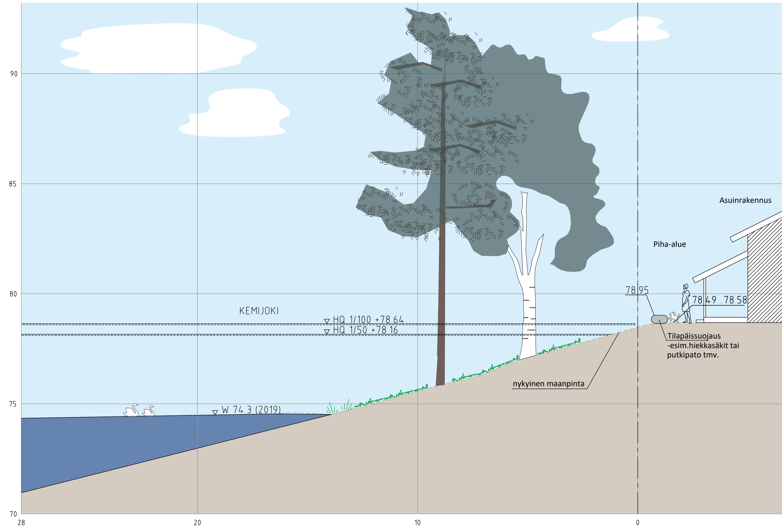
Leikkaus Kulpinranta PL120 / Kulpinranta 9-11 1:100
